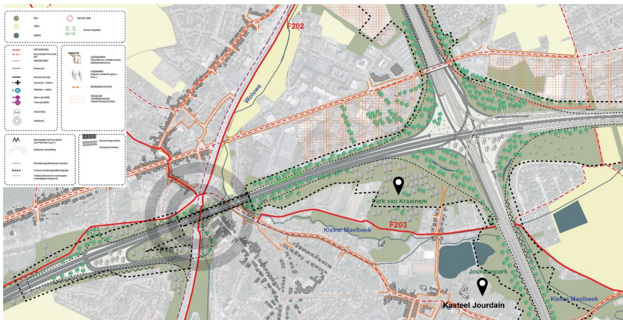
Figure 123: Échangeur R0/E40 - Woluwe-Saint-Étienne variante G2a' (Cycle 2)
