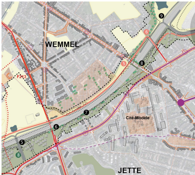
Figure 35 : Développement spatial du profil longitudinal optimisé a avec passages souterrains Zone Wemmel-Jette - Cycle 2 (LPa_WM)
