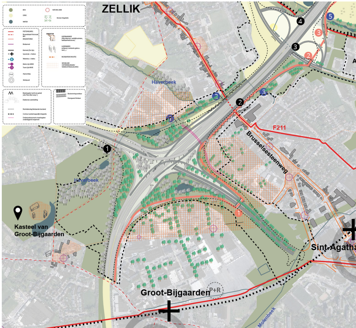
Figure 107 : Échangeur R0/E40 Grand-Bigard, variante G1a (Cycle 2)
