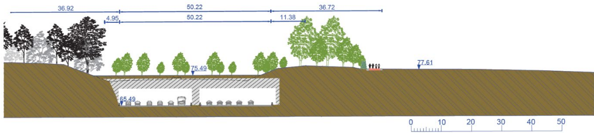
Figure 32 : coupe transversale B - G1 LPb_LB
