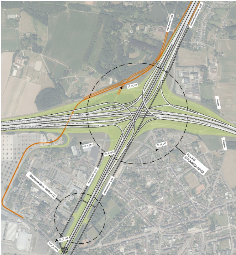
Figure 65 : échangeur /nœud A12 Strombeek-Bever variante a' dans G2- Cycle 2 → avec variante nœud en étoile 4/4 RU
