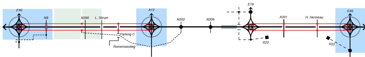
Figure 144 : Diagramme linéaire de l'alternative du cycle 2 - G2a
