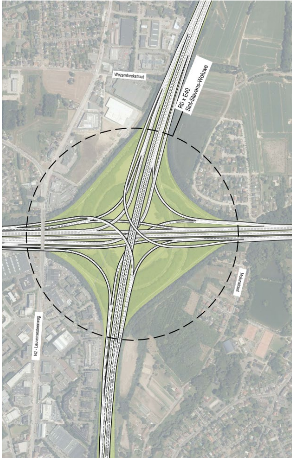
Figure 70 : échangeur R0/E40 Woluwe-Saint-Étienne variante a' dans G2 - Cycle 2 → nœud en étoile 4/4 RU
