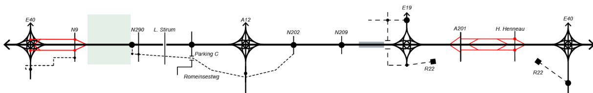
Figure 141 : Diagramme linéaire de l'alternative du cycle 2 - G1a avec LPb-LB
