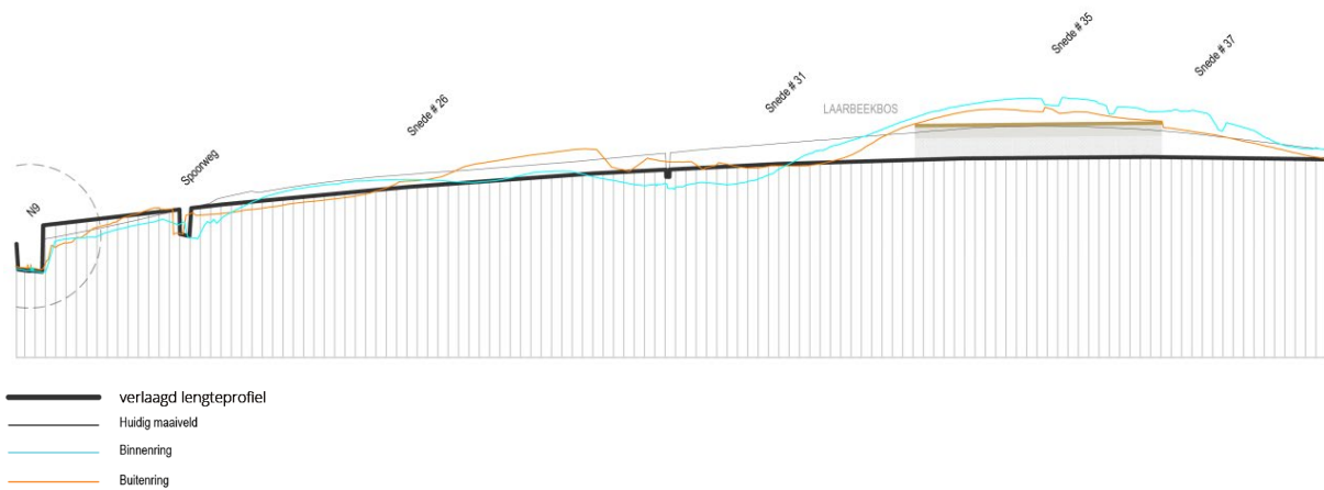
Figure 27 : Profil longitudinal abaissé a avec un pont paysager maximal - (Cycle 2) (profil longitudinal mis à l'échelle 5x par rapport à la hauteur de l'axe Y)
