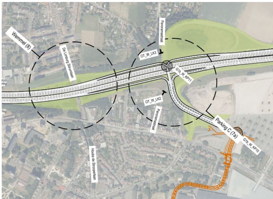
Figure 75: Complexe de raccordement 7a – Parking C dans G1 - Cycle 2 (la situation de référence est en orange)
