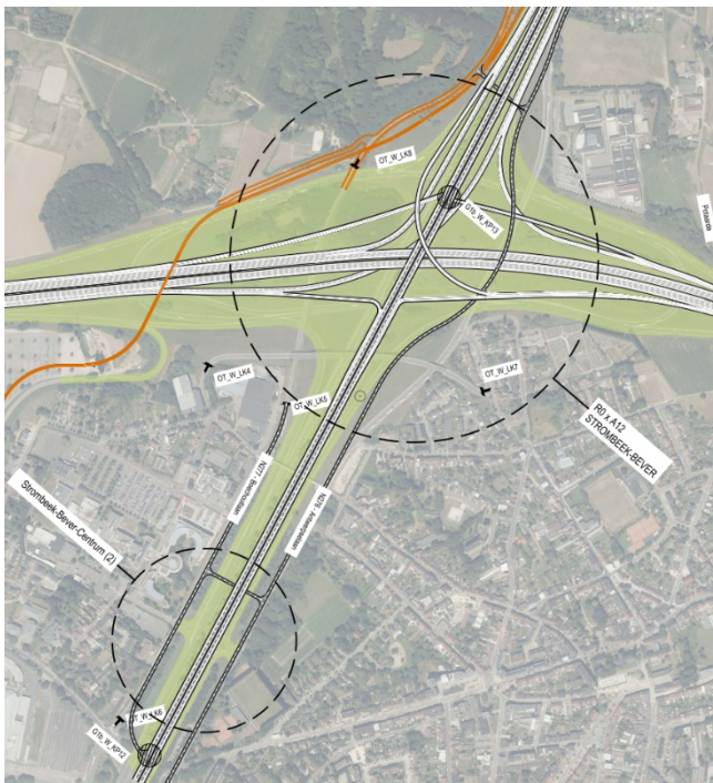
Figure 53 : échangeur /nœud A12 Strombeek-Bever dans G1b- Cycle 2 → avec variante nœud en étoile 3/4
