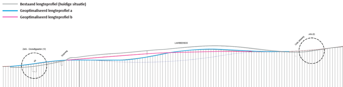
Figure 20 : Étude du profil longitudinal de la sous-zone du Bois du Laerbeek (où le profil longitudinal est mis à l'échelle 5x par rapport à la hauteur de l'axe Y)
