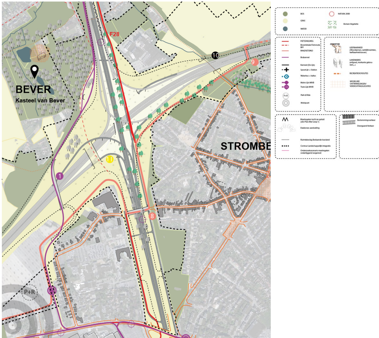
Figure 109 : Échangeur R0/A12 Strombeek-Bever variante G1a (Cycle 2)
