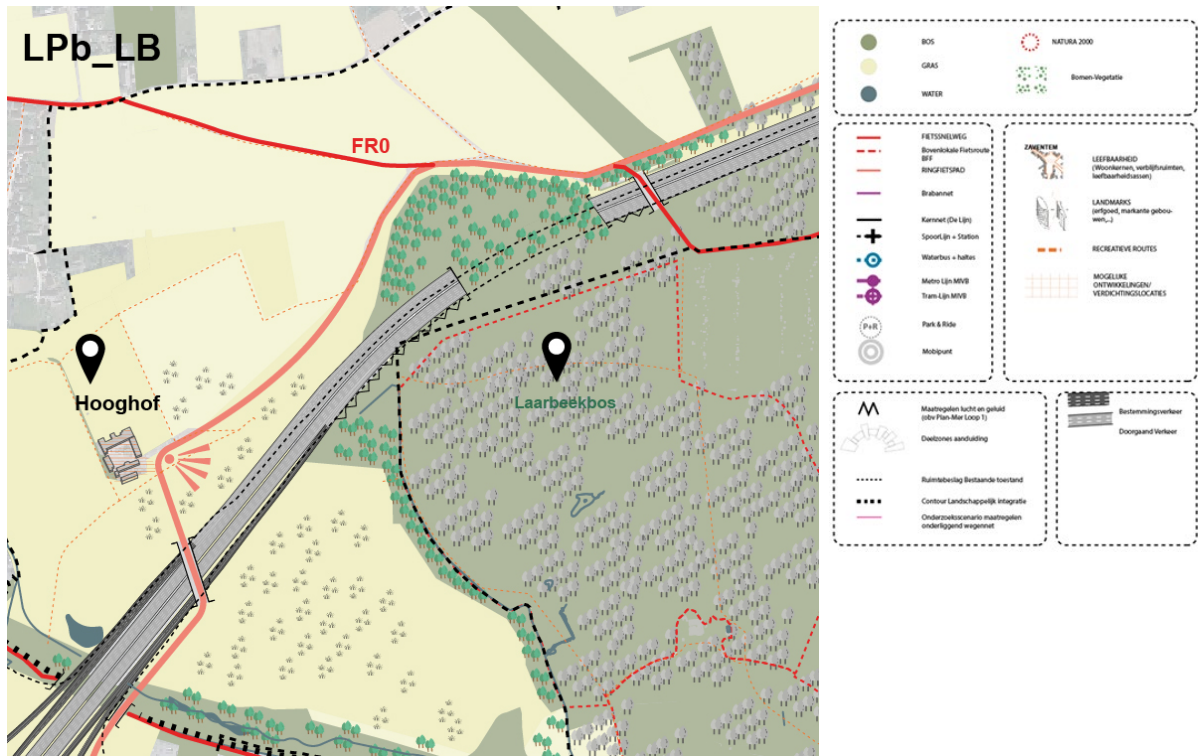
Figure 126 : Profil longitudinal optimisé b avec un pont paysager maximal (LPb LB) sous-zone du Bois du Laerbeek (illustration pour l'alternative 1)
