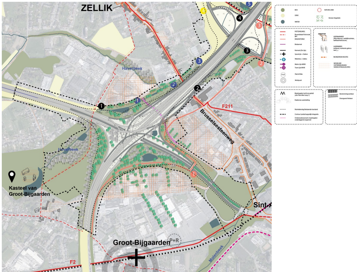
Figure 116 : Échangeur R0/E40 Grand-Bigard, variante G2a (Cycle 2)
