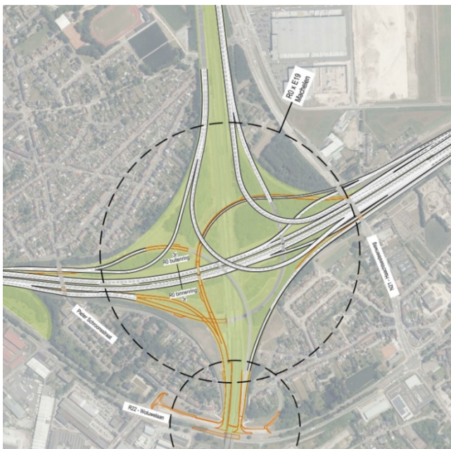
Figure 67 : échangeur /nœud E19 Machelen dans G2 - cycle 2 → avec un nœud en étoile 4/4 RU
