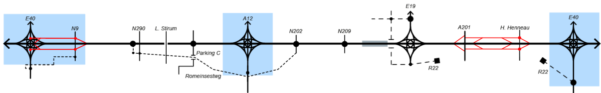
Figure 105 : Diagramme linéaire de l'Alternative 1 avec nœuds symétriques 4/4 (G1a)
