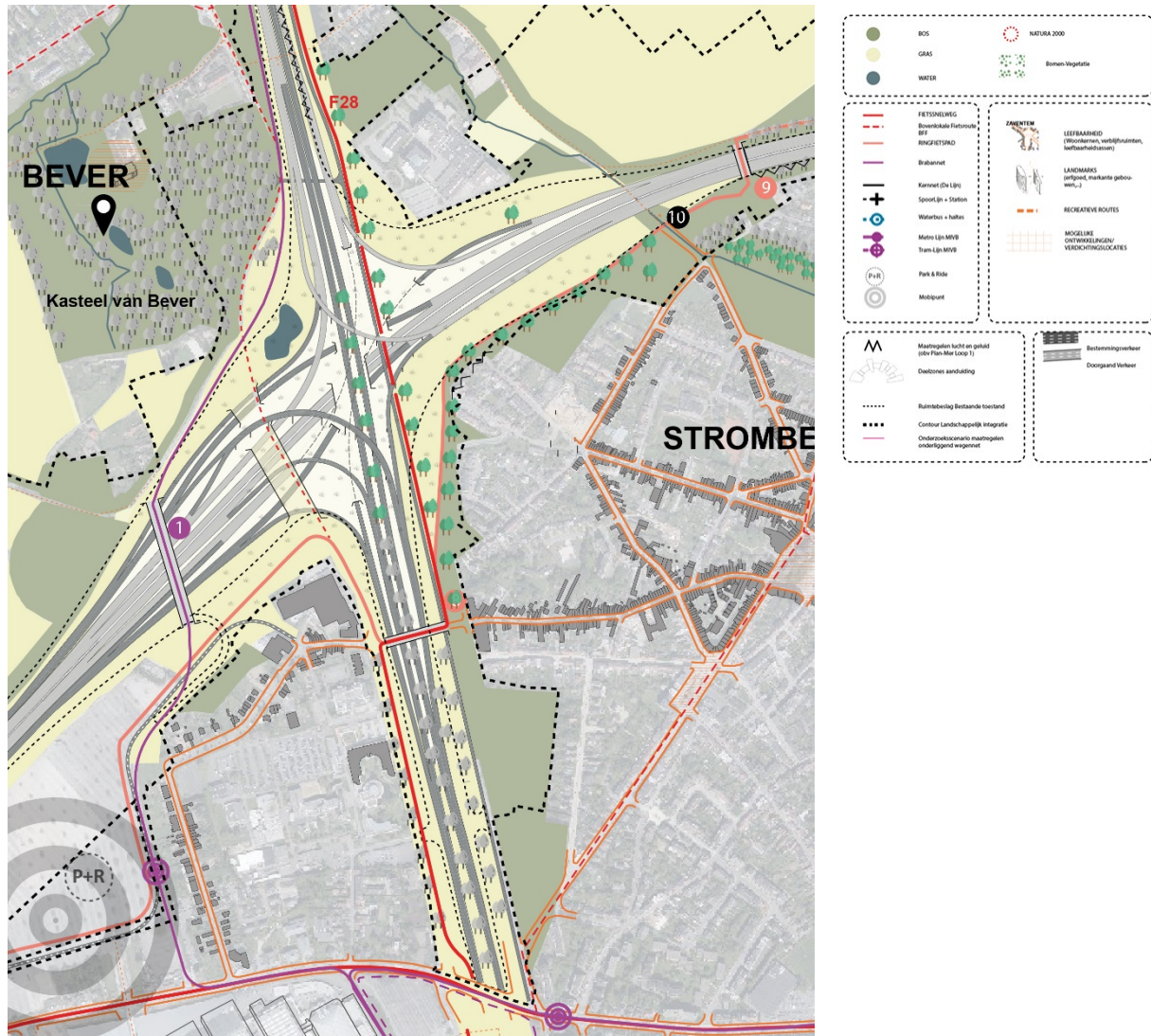
Figure 120 : Échangeur R0/A12 Strombeek-Bever variante G2a' (cycle 2)
