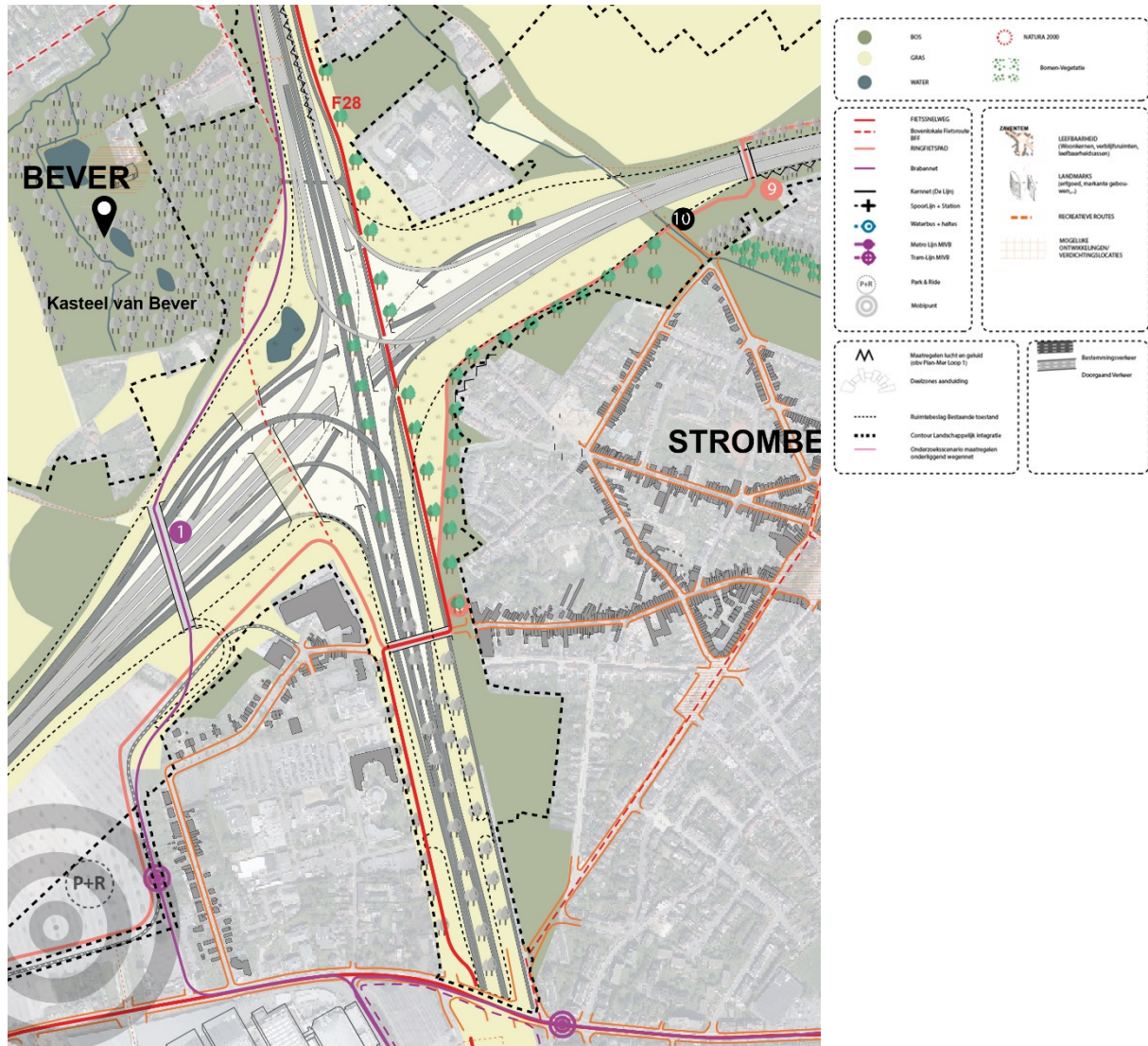
Figure 119 : Échangeur R0/A12 Strombeek-Bever variante G2a (Cycle 2)
