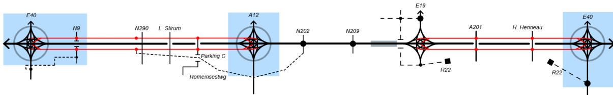
Figure 113 : Diagramme linéaire de l'Alternative 2 avec nœuds symétriques 4/4 sur le RU et le RC (G2a)
