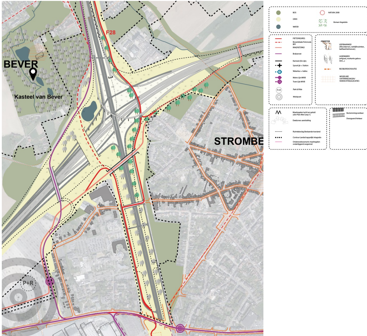
Figure 121 : Échangeur R0/A12 Strombeek-Bever variante G2b (Cycle 2)
