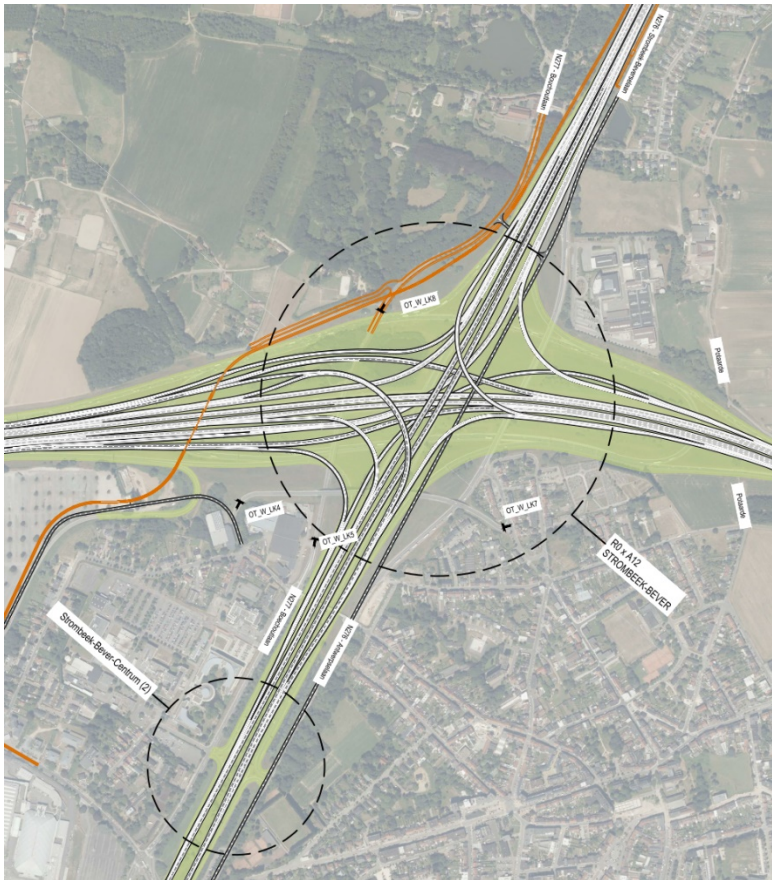
Figure 64 : échangeur A12 Strombeek-Bever variante a dans G2- Cycle 2 → avec variante nœud en étoile 4/4 RU et RC
