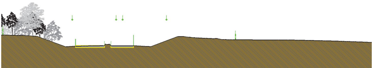
Figure 25 : Coupe transversale BB - situation existante
