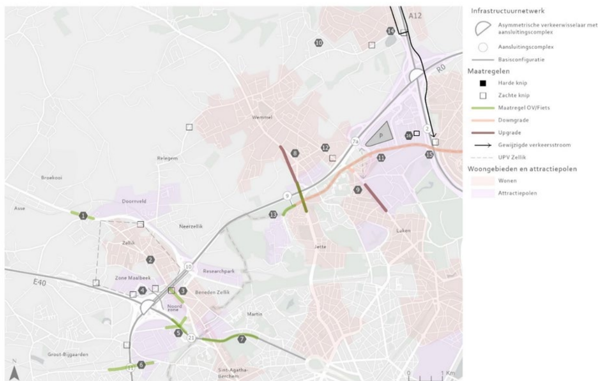
Figure 135 : Zone Wemmel - Indication des mesures sur le réseau routier secondaire
