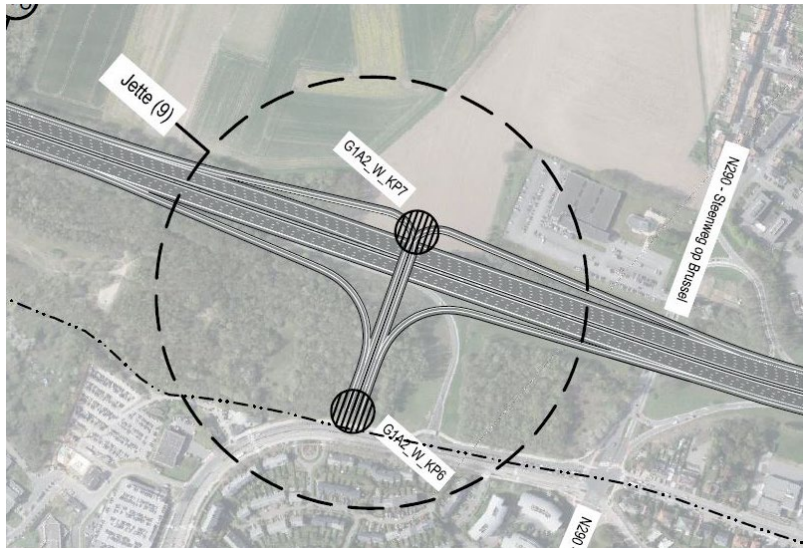
Figure 72: Complexe de raccordement 9 Jette/N290 dans G1A2 - cycle 1
