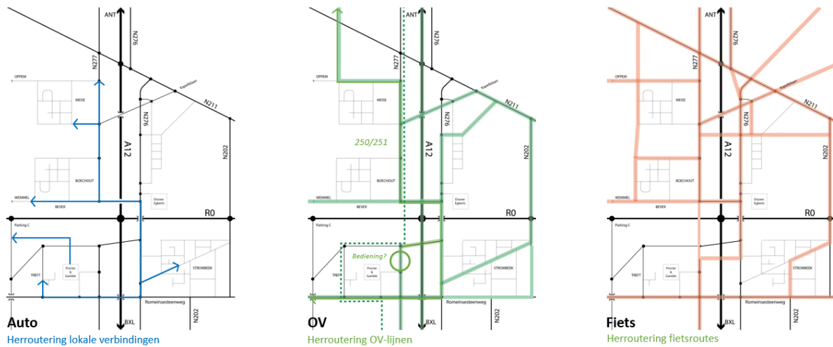
Figure 83 : Représentation schématique du désenclavement des environs de l'A12 - alternative G2a
