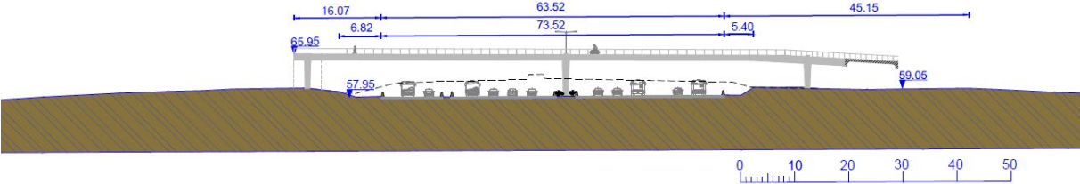
Figure 30 : coupe transversale A - G1 LPb_LB
