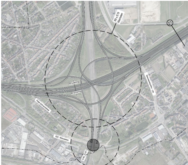
Figure 54 : échangeur /nœud E19 Machelen dans G1A2 - Cycle 1 avec un nœud 4/4
