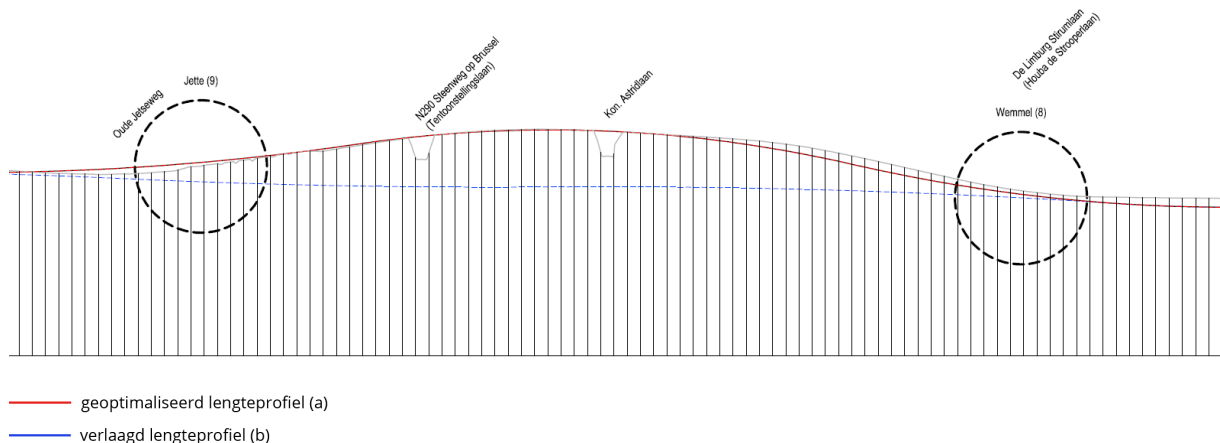
Figure 33 : Étude du profil longitudinal de la sous-zone de Wemmel-Jette (le profil longitudinal mis à l'échelle 5x par rapport à la hauteur de l'axe Y)
