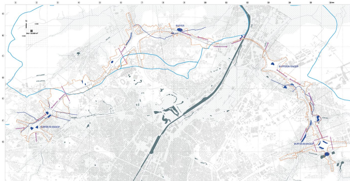
Figure 90 : Vision de l'évacuation des eaux et des bassins tampons étude conceptuelle - Cycle 2 le long de R0-Nord
