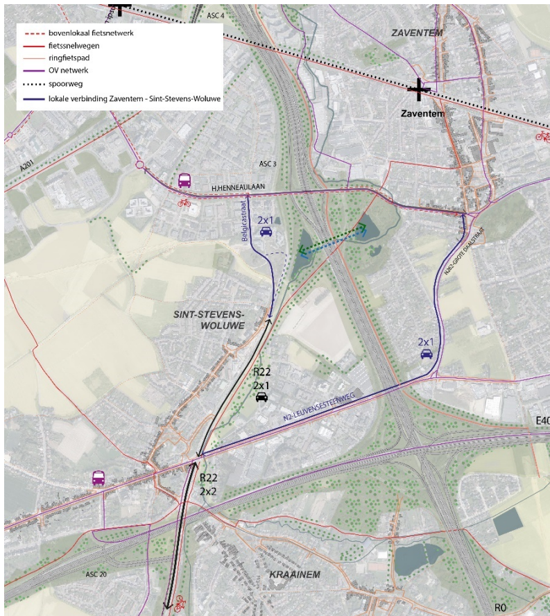
Figure 137 : Mesures sur le réseau routier secondaire dans la zone de Zaventem - connexion locale via la R22
