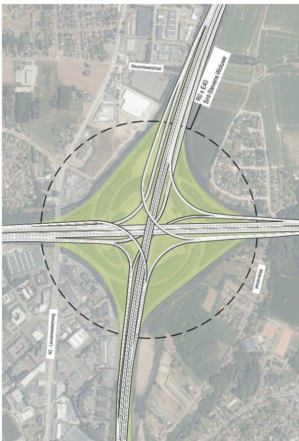
Figure 57 : échangeur /nœud E40 Woluwe-Saint-Étienne dans G1 - cycle 2 → avec un nœud en étoile 4/4
