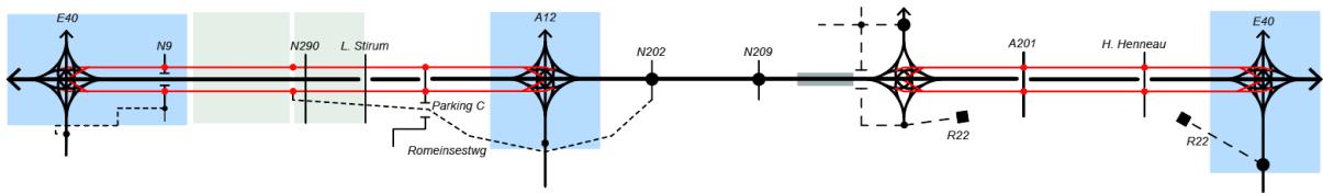
Figure 104 : Diagramme linéaire de l'alternative 2 avec éléments variables
