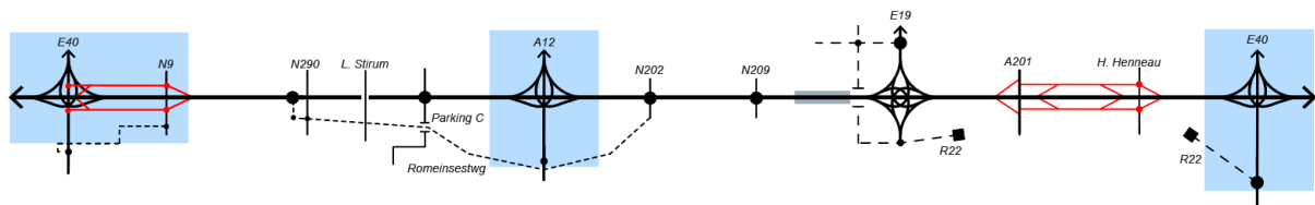
Figure 106 : Diagramme linéaire de l'Alternative 1 avec nœuds asymétriques 3/4 (G1b)
