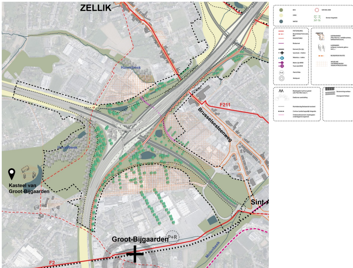
Figure 118 : Échangeur R0/E40 Grand-Bigard, variante G2b (Cycle 2)
