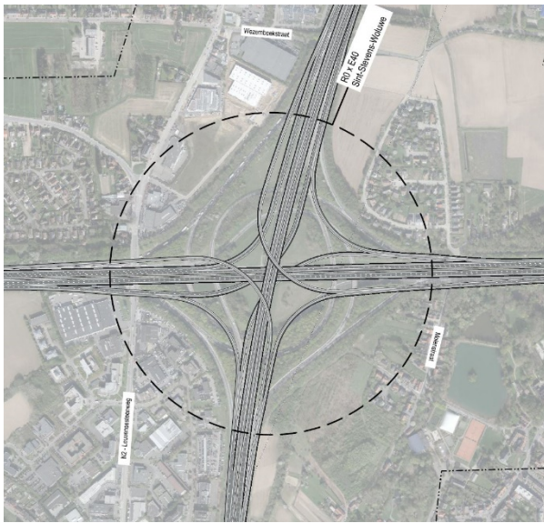
Figure 56 : échangeur /nœud E40 Woluwe-Saint-Étienne dans G1A2 - Cycle 1 avec un nœud 4/4
