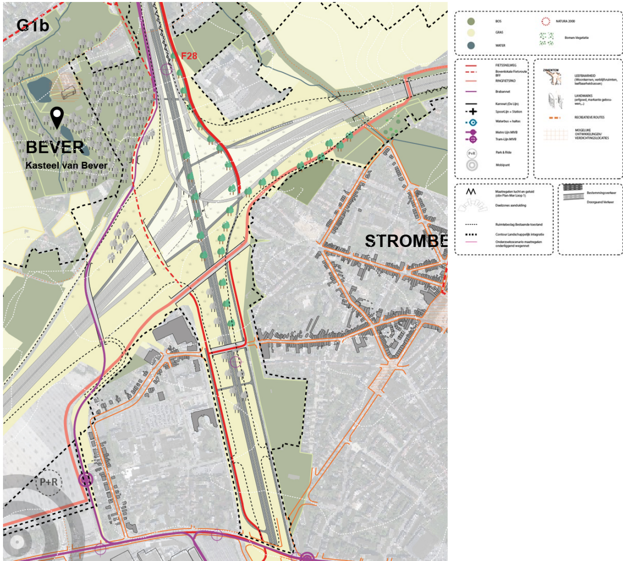
Figure 110 : Échangeur R0/A12 Strombeek-Bever variante G1b (Cycle 2)
