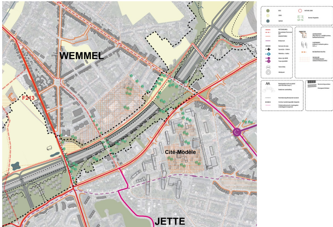
Figure 128 : Profil longitudinal abaissé b avec pont du R0-Nord (LPb_WM1) sous-zone de Wemmel-Jette (illustration pour l'alternative 2)
