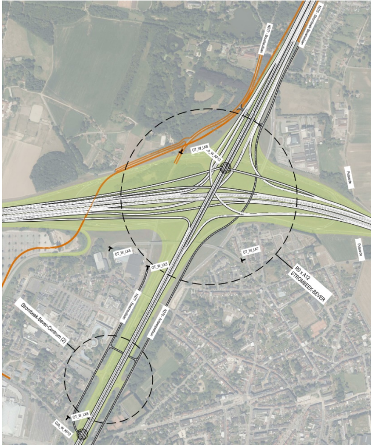
Figure 66 : échangeur /nœud A12 Strombeek-Bever variante b dans G2- Cycle 2 → avec variante nœud 3/4 RU
