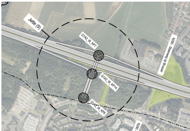
Figure 73: Complexe de raccordement 9 Jette/N290 dans G1 - cycle 2
