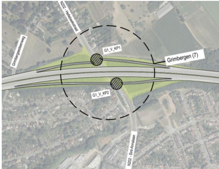
Figure 76: Complexe de raccordement 7 – Grimbergen/ N202 dans G1 – Cycle 2
