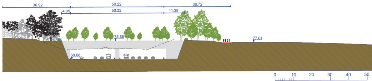
Figure 26 : coupe transversale BB - G1 LPa_LB
