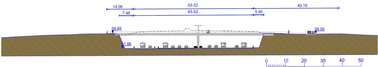
Figure 24 : coupe transversale AA - G1 LPa_LB
