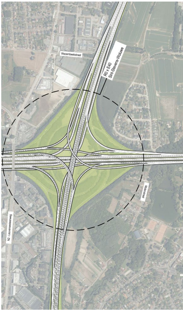
Figure 69 : échangeur R0/E40 Woluwe-Saint-Étienne variante a dans G2 - Cycle 2 → nœud en étoile 4/4 RU et RC
