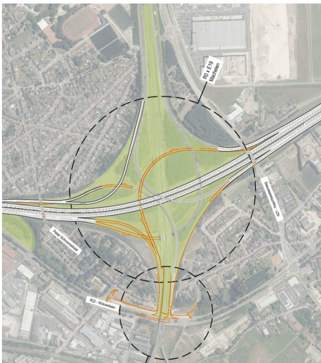
Figure 55 : échangeur /nœud E19 Machelen dans G1 - Cycle 2 → avec un nœud en étoile 4/4
