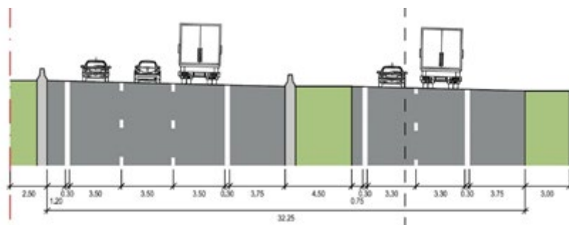
Figure 15 : Principe du profil G2 (alternative parallèle) - cycle 1 avec accotements centraux
