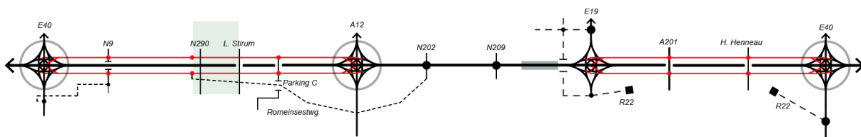
Figure 149 : Diagramme linéaire de l'alternative du cycle 2 - G2a avec LPb-WM-2
