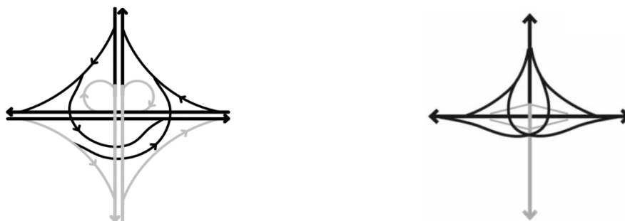
Figure 143 : Représentation schématique de l'échangeur asymétrique à quatre bras (à gauche, aérien, à droite, au niveau du sol) - (en gris, le boulevard de Bruxelles)
