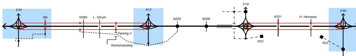
Figure 160 : Diagramme linéaire de l'Alternative 2 avec nœuds asymétriques 3/4 sur le RU
