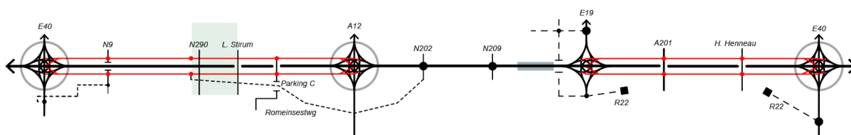
Figure 180 : Diagramme linéaire de l'alternative 2 du Cycle 2 - G2a avec LPb-WM-2
