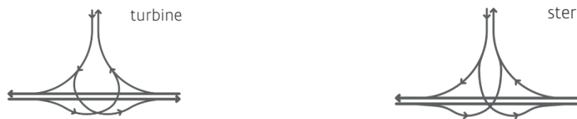
Figure 142 : Représentation schématique d'un échangeur à trois bras
