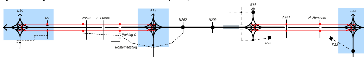
Figure 159 : Diagramme linéaire de l'Alternative 2 avec nœuds symétriques 4/4 sur le RU
