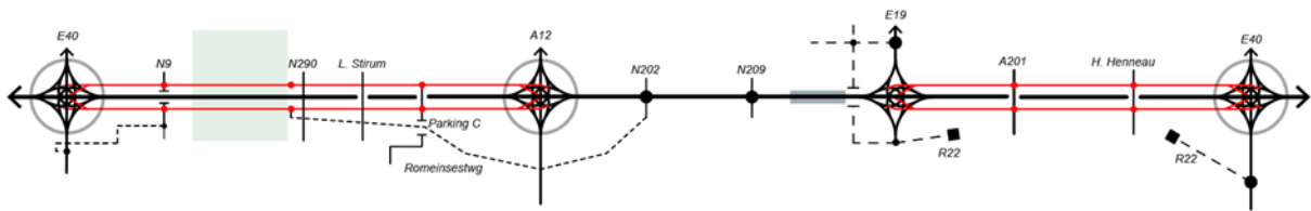
Figure 177 : Diagramme linéaire de l'alternative 2 du Cycle 2 - G2a avec LPa-LB-2
