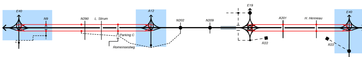
Figure 176 : Diagramme linéaire de l'alternative 2 du Cycle 2 - G2b
