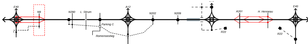
Figure 171: Schéma linéaire de l'alternative 1 du Cycle 2 - G1a avec CR 10 comme complexe hollandais
