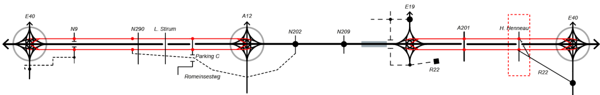
Figure 183 : Schéma linéaire de l'alternative 2 Cycle 2 - G2a avec indication de la variante R22
