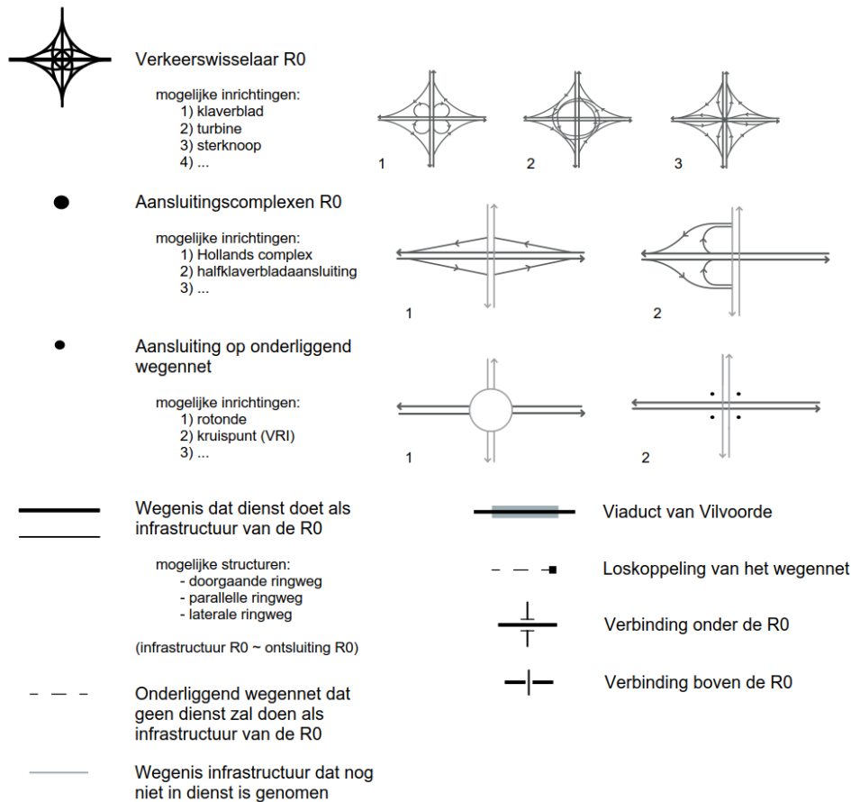
Figure 131 : Légende des schémas linéaires des alternatives raisonnables distinctes Groupe 1 - Light
