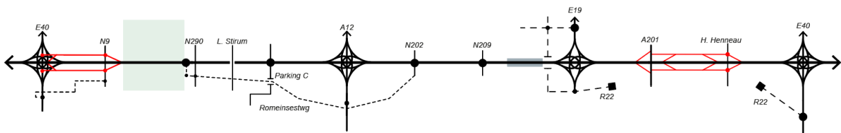
Figure 168 : Diagramme linéaire de l'alternative 1 du Cycle 2 - G1a avec LPb-LB
