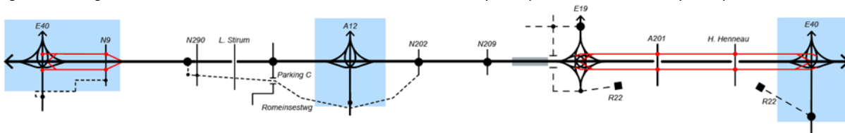
Figure 163 : Diagramme linéaire de l'Alternative 3 avec nœuds asymétriques 3/4
