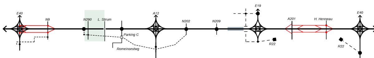
Figure 170 : Diagramme linéaire de l'alternative 1 du Cycle 2 - G1a avec LPb-WM-2
