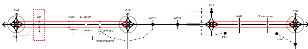
Figure 181: Schéma linéaire de l'alternative 2 du Cycle 2 - G2a avec CR 10 comme complexe hollandais
