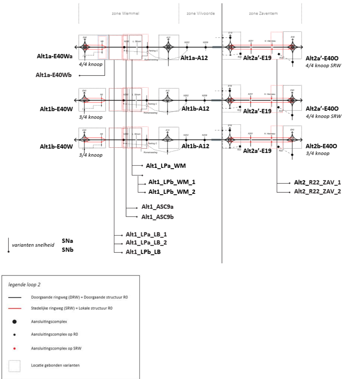
Figure 184 : Diagrammes linéaires de l'alternative 3 et de ses variantes dans le Cycle 2
