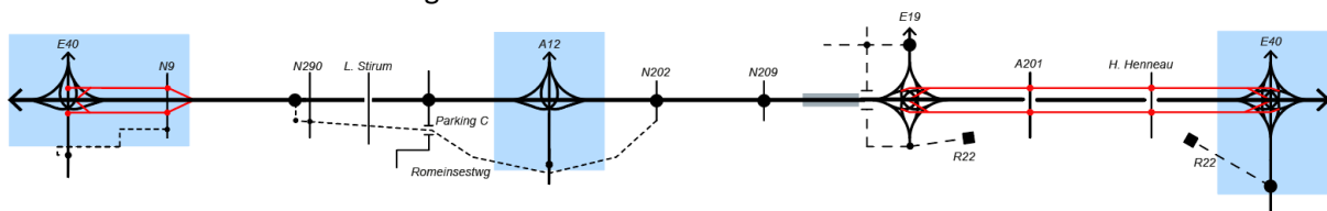
Figure 186 : Diagramme linéaire de l'alternative 3 du Cycle 2 - G1b/G1b/G2a'
