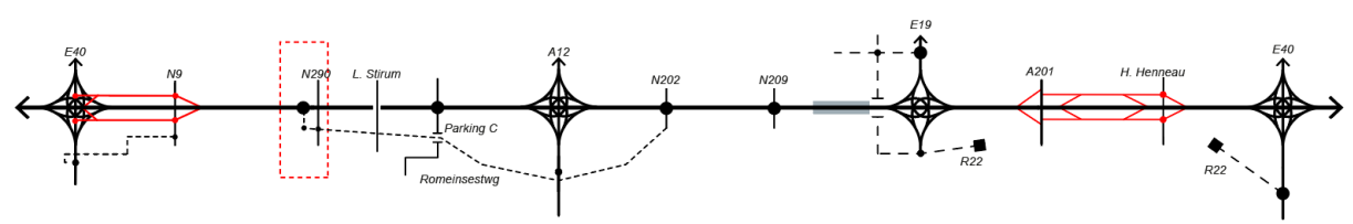
Figure 172 : Schéma linéaire de l'alternative 1 du Cycle 2 – G1a avec CR 9 comme SPI
