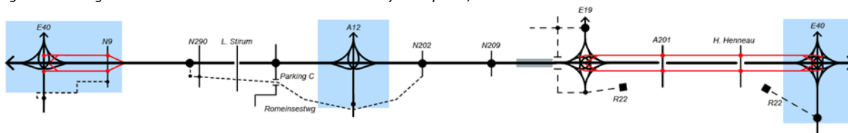
Figure 162 : Diagramme linéaire de l'alternative 3 avec combinaison de nœuds symétriques 4/4 et d'un nœud asymétrique 4/4
