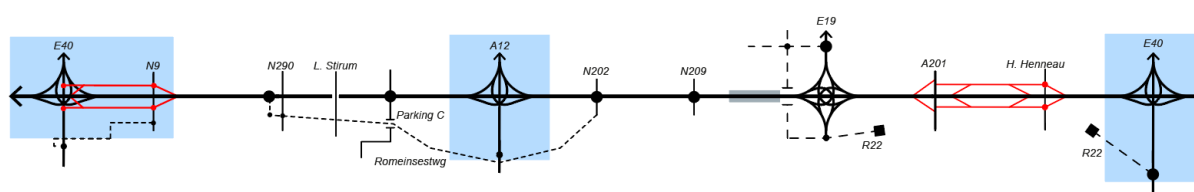
Figure 157 : Diagramme linéaire de l'Alternative 1 avec nœuds asymétriques 3/4
