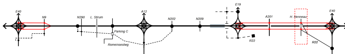
Figure 194 : Schéma linéaire G1aG1aG2a' avec indication de la variante R22
