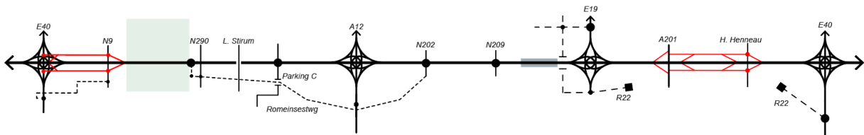
Figure 167 : Diagramme linéaire de l'alternative 1 du Cycle 2 - G1a avec LPa-LB-2
