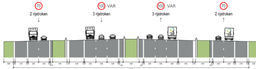
Figure 125 : Profil transversal de type G2 - parallèle
