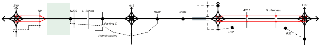
Figure 188 : Schéma linéaire G1aG1aG2a' avec indication de la variante Lpa_LB_2
