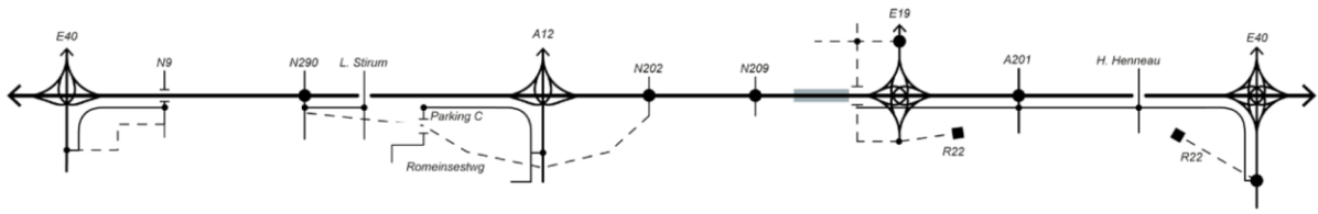
Figure 137 : Diagramme linéaire de l'alternative raisonnable distincte G3A2
