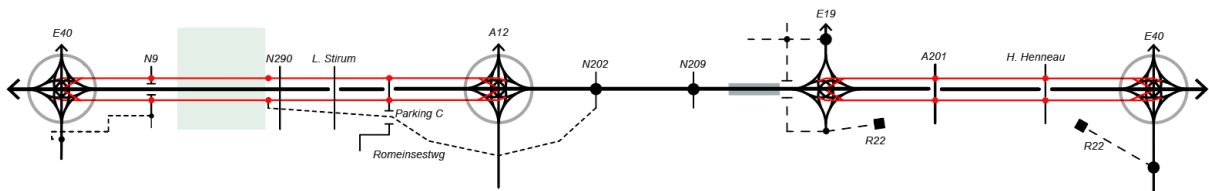
Figure 178 : Diagramme linéaire de l'alternative 2 du Cycle 2 - G2a avec LPb-LB
