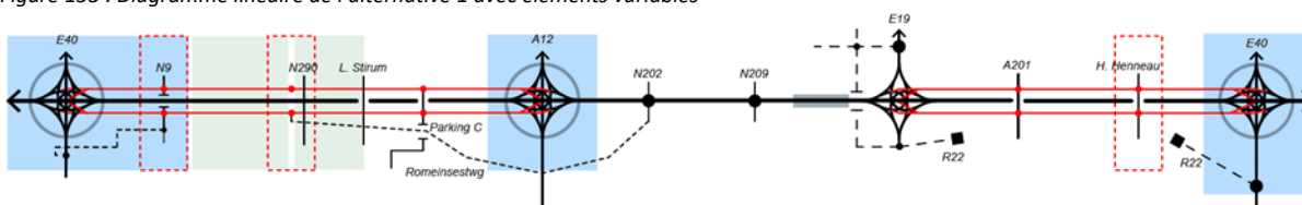
Figure 154 : Diagramme linéaire de l'alternative 2 avec éléments variables
