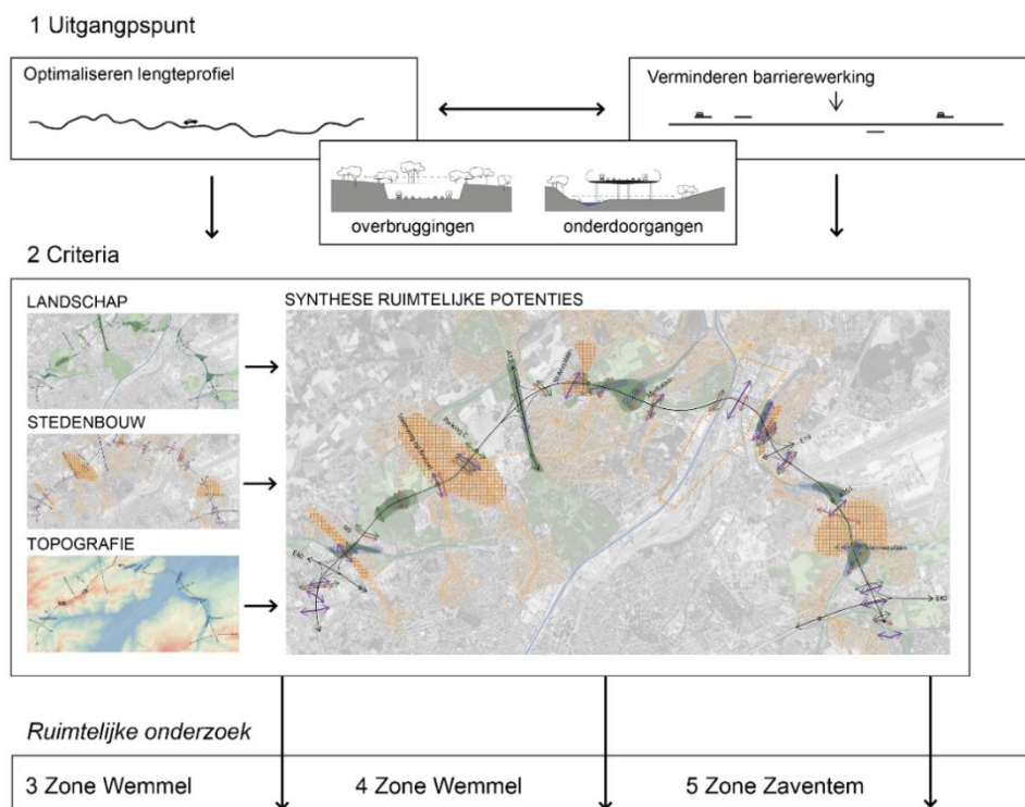
Figure 145 : Représentation schématique de la méthodologie de l'étude du profil longitudinal La description détaillée est fournie à l'annexe 5 (« Étude des variantes raisonnables du Cycle 1 »).
