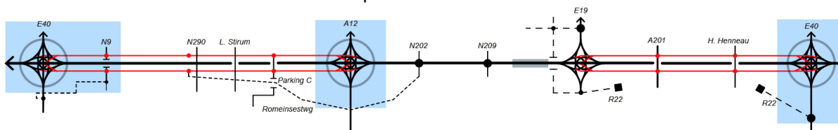
Figure 158 : Diagramme linéaire de l'Alternative 2 avec nœuds symétriques 4/4 sur le RU et le RC
