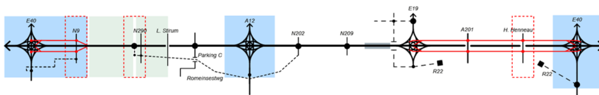
Figure 161 : Diagramme linéaire de l'Alternative 3 avec nœuds symétriques 4/4
