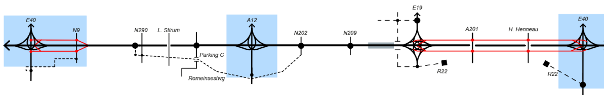
Figure 187 : Diagramme linéaire de l'alternative 3b du Cycle 2 - G1b/G1b/G2b
