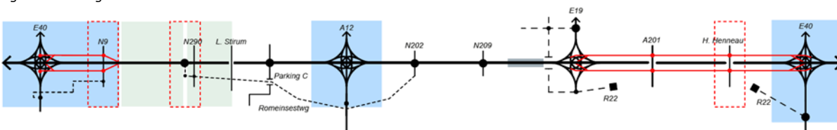
Figure 155 : Diagramme linéaire de l'alternative 3 avec éléments variables
