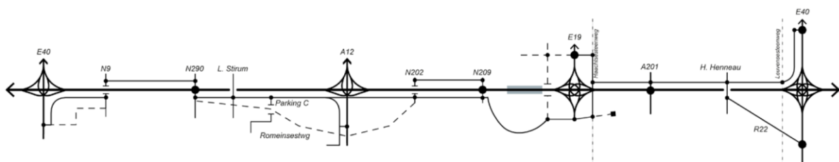
Figure 136 : Diagramme linéaire de l'alternative raisonnable distincte G3A1
