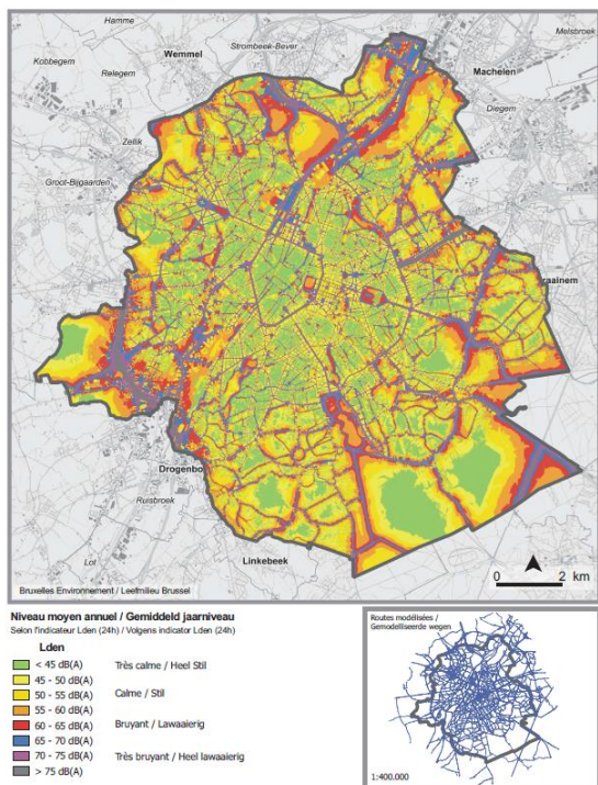
Figure 202 : Carte du bruit de la circulation routière Lden à proximité de la zone du plan - année de référence 2016 (source : Bruxelles Environnement (IGBE).
